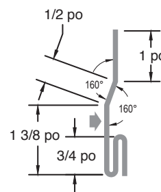
Départ général 352
