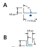
350 Couvre-joints A et B en deux pièces
