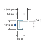
313 Couvre-joint en J
