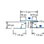
321 Moulure de cloison
